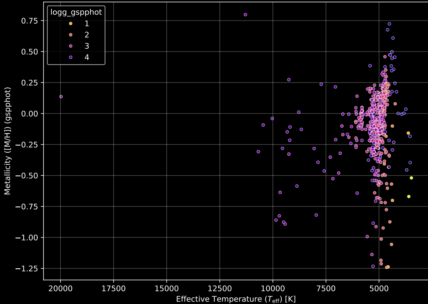
APOGEE DR17 Field: [120+08] Stellar Population Parameters (n= 561)
